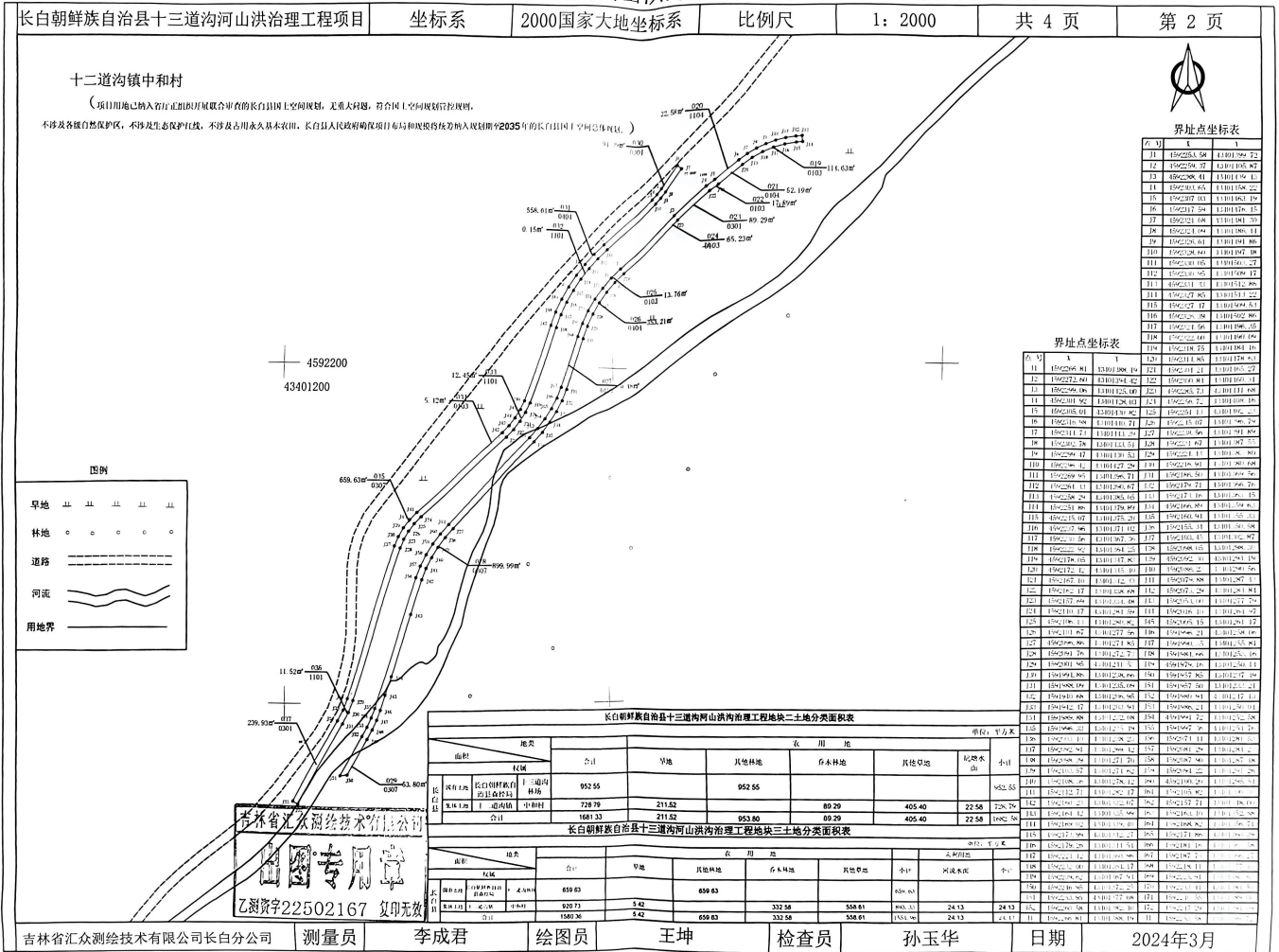
长白朝鲜族自治县十三道沟河山洪沟治理工程项目用地勘测定界技术图
